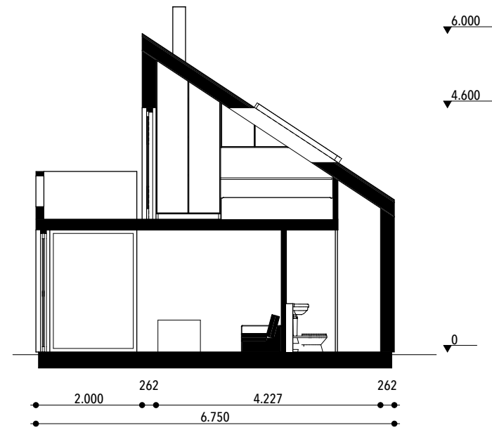
Doorsnede C-C
