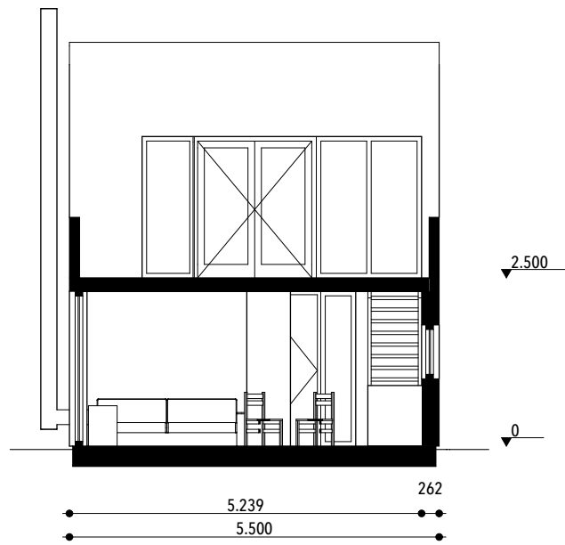
Doorsnede B-B
