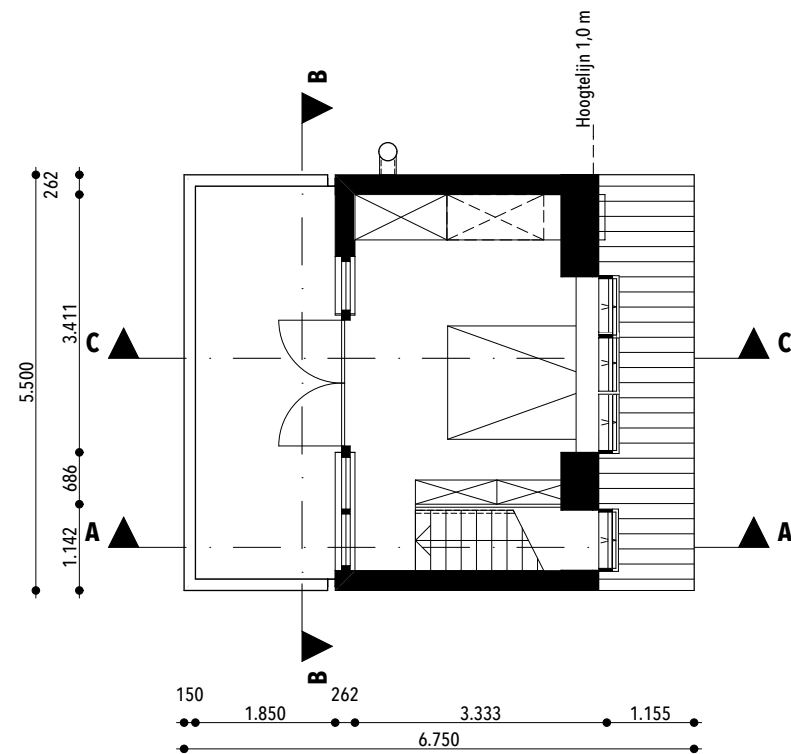
Plattegrond eerste verdieping
