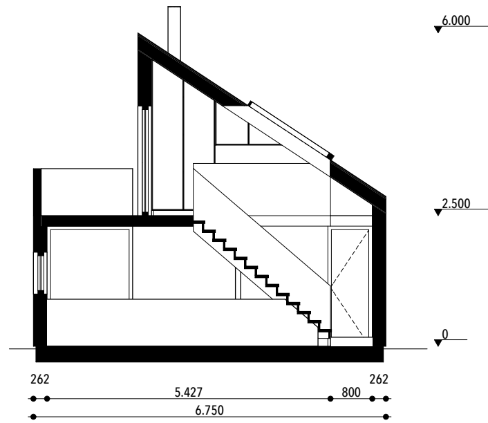
Doorsnede A-A
